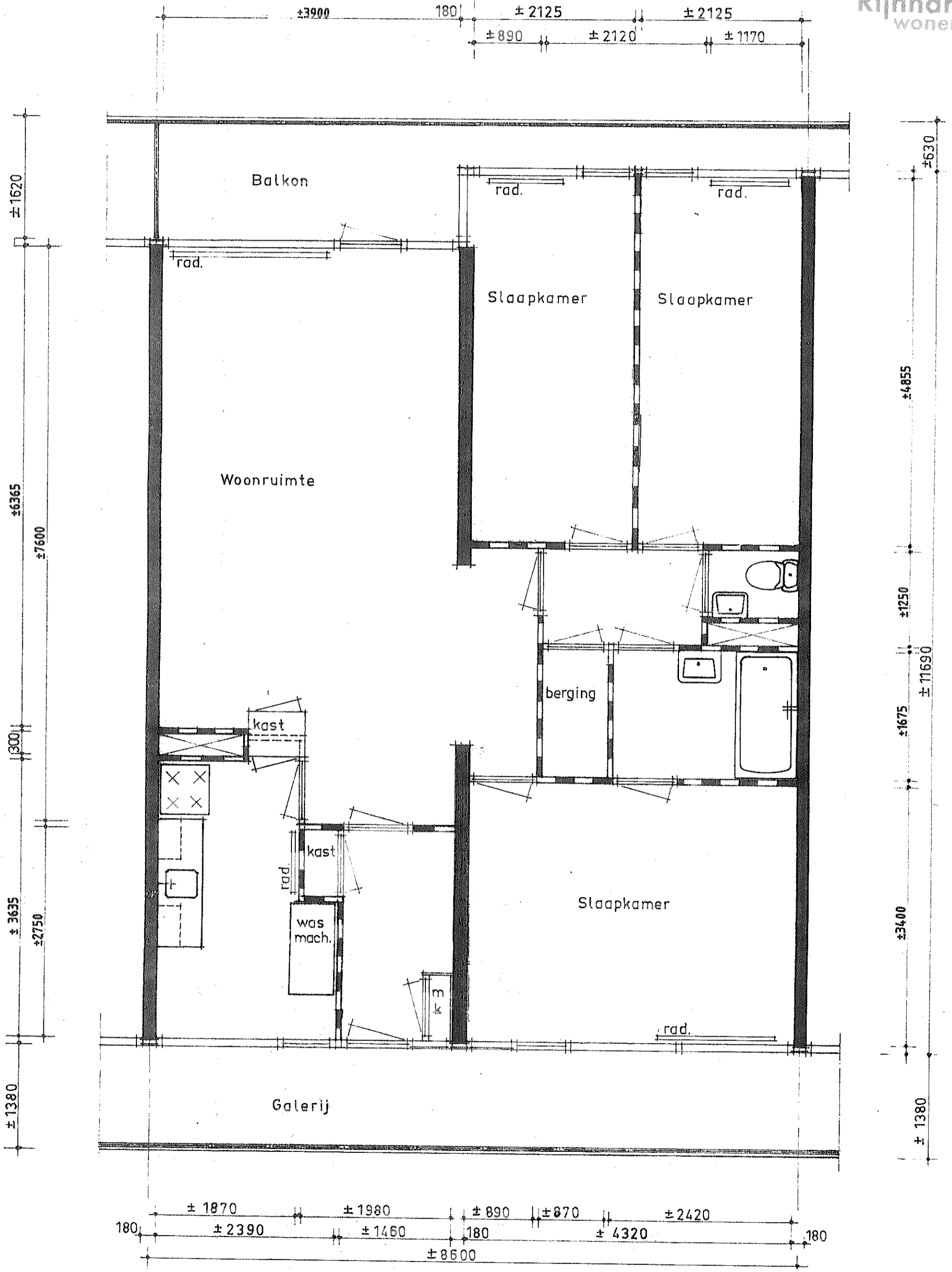
Plattegrond 1:50
